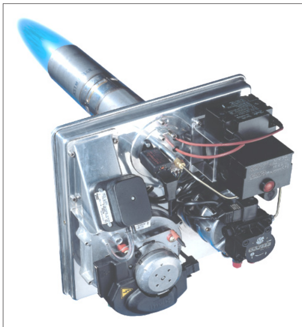
Blaubrenner Blautherm DUO der Scheer Heizsysteme & Produktionstechnik GmbH, Wöhrden
